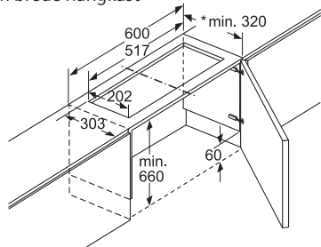
Montage toestel met cleanAir-module en neerlaatkader
