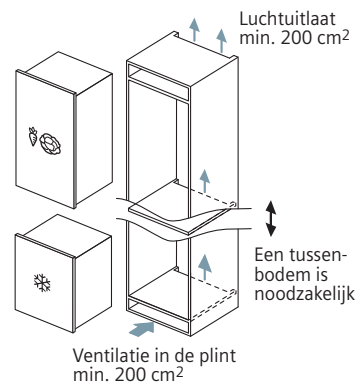
modularFit - Verticale combinatie
