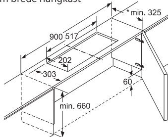
Montage toestel met cleanAir-module en neerlaatkader
