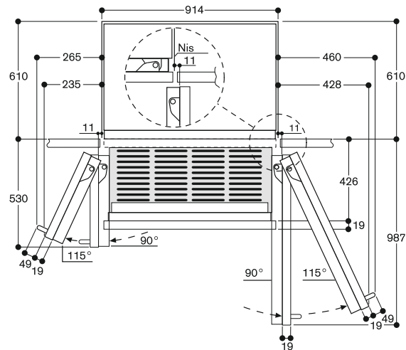
In de tekening wordt uitgegaan van een meubelfrontdikte van 19 mm alsmede de hoogte van een Gaggenau meubelgreep van 49 mm.
