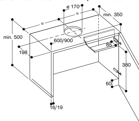
Bovenkast voor AF 210/211 met verzinkbaar kader AA 210 460 / AA 210 490
