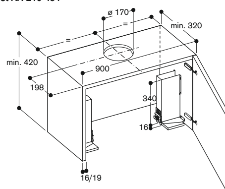
Bovenkast voor AF 210/211 met AA 210 491
