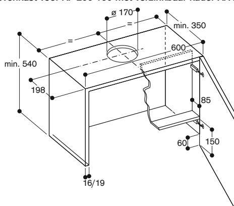
Bovenkast voor AF 200 160 met verzinkbaar kader AA 210 460
