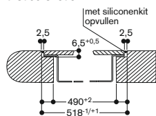
Dwarsdoorsnede
