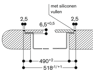
Dwarsdoorsnede
