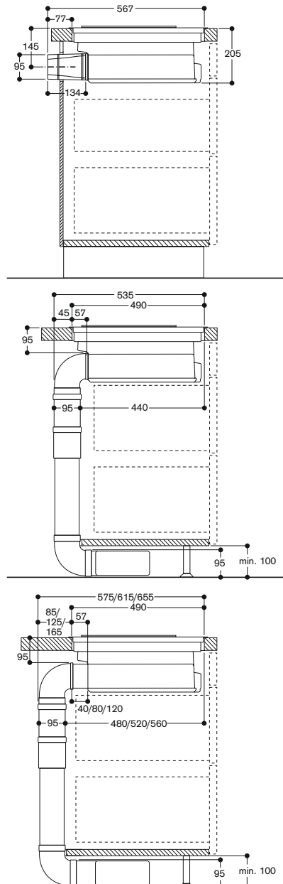
Zijaanzicht CV 282 met platte buis-aansluitstuk CA 284-010
