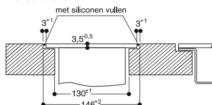
Dwarsdoorsnede
