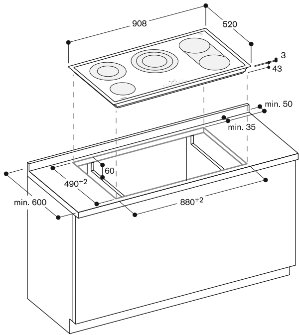
Nisdiepte in de nabijheid van de elektrische aansluitingsdoos: 65 mm.
