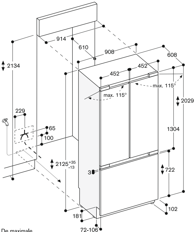
De maximale deurfrontafmetingen zijn gedimensioneerd voor een spleetmaat van 3 mm.
