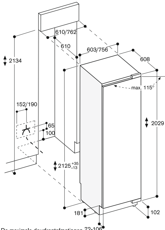
De maximale deurfrontafmetingen 72-106 zijn gedimensioneerd voor een spleetmaat van 3 mm.
