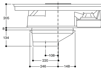
Vooraanzicht CV 282 met platte buis-aansluitstuk CA 284-010
