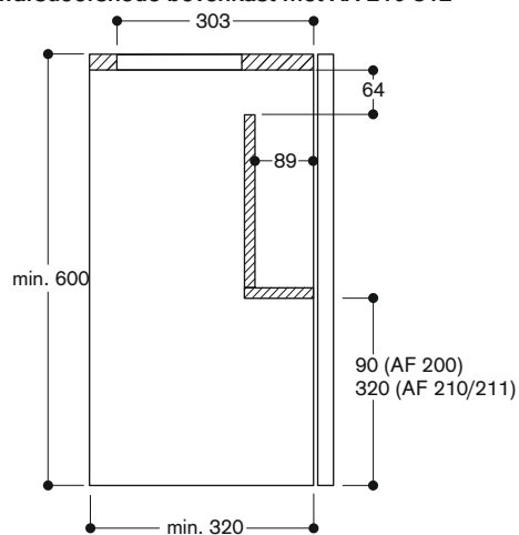
Dwarsdoorsnede bovenkast met AA 210 812
