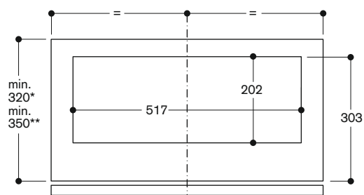
Aanzicht bovenkast van boven met AA 210 812
