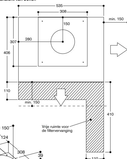
Aanzicht van boven
