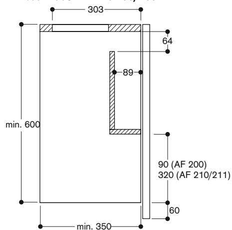
Dwarsdoorsnede bovenkast met AA 210 812 en verzinkbaar kader AA 210 490/460
