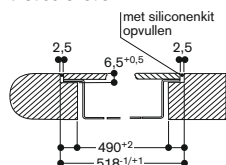
Dwarsdoorsnede
