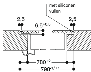
Lengte doorsnede
