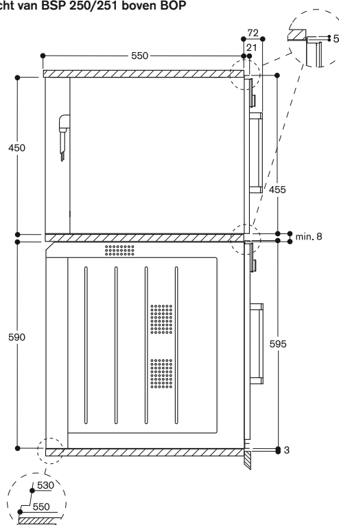
Zijaanzicht van BSP 250/251 boven BOP
