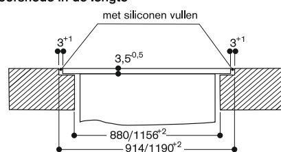
Doorsnede in de lengte
