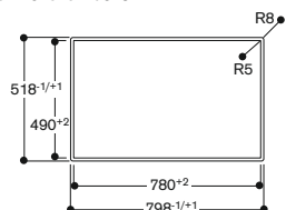
Aanzicht van boven
