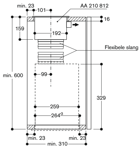
Dwarsdoorsnede bovenkast met AC 200 en AA 210 812
