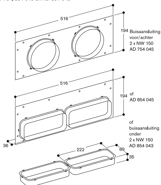
AD 754/854 045 en AD 854 043
