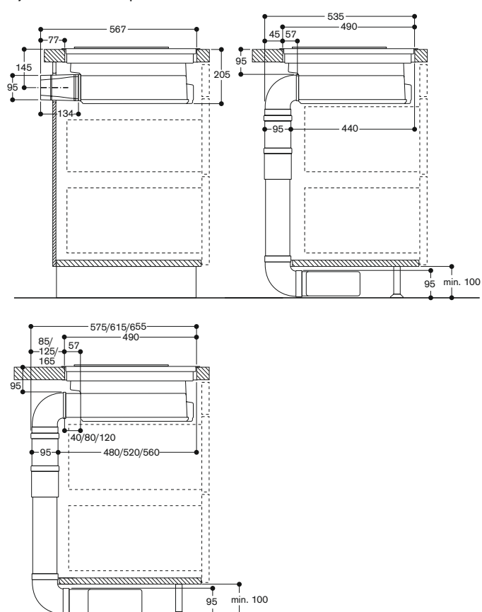
Zijaanzicht CV 282 met platte buis-aansluitstuk CA 284-010
