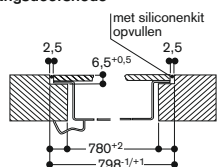
Langsdoorsnede
