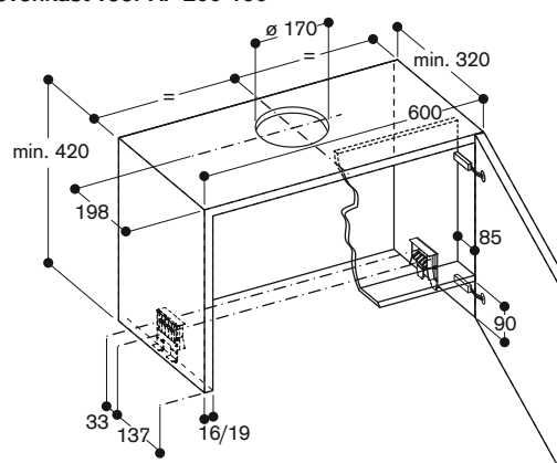
Bovenkast voor AF 200 160
