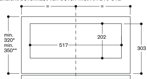
Aanzicht bovenkast van boven met AA 210 812
