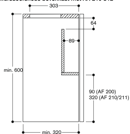
Dwarsdoorsnede bovenkast met AA 210 812
