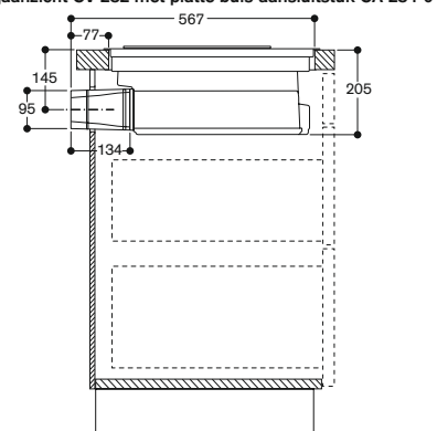
Zijaanzicht CV 282 met platte buis-aansluitstuk CA 284-010
