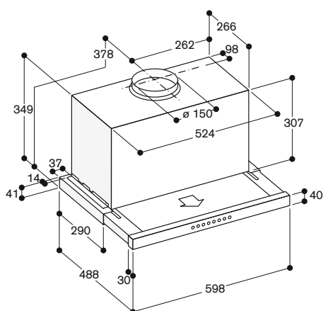
Bovenkast voor AF 210/211
